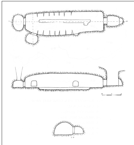
FIGURA 1.- Planta i seccions hipogeu d'en Miquel Bordoy (Bordoy, 1945)
