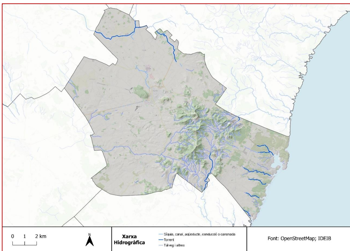
Figura 7. Mapa de la hidrologia superficial del terme municipal de Felanitx. Alguns dels torrents més importants que discorren dintre dels límits del municipi són: torrent de Son Valls, torrent de Son Cifre, torrent de de Ca
