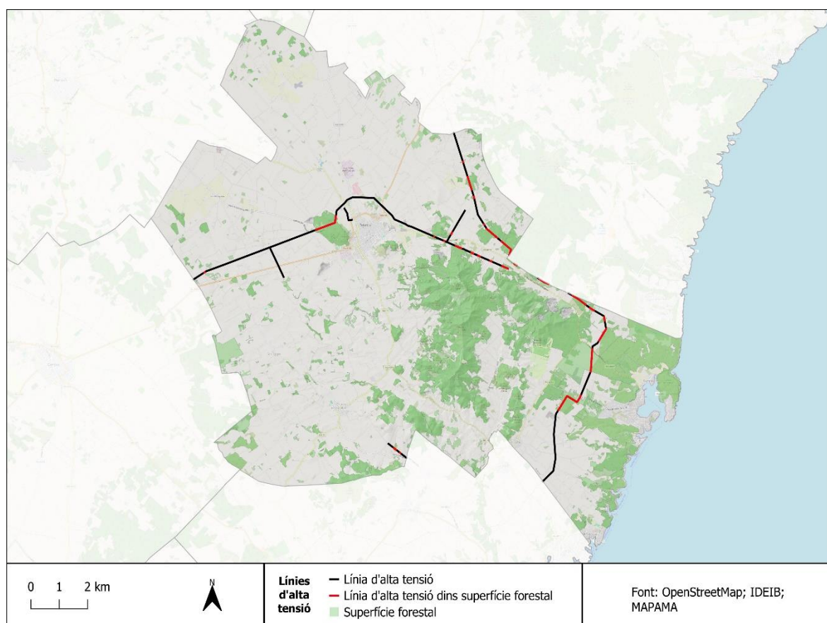
Figura 24. Línies d'alta tensió del municipi de Felanitx ressaltant els trams ubicats dins zona forestal. Font: Elaboració pròpia a partir de OSM i MAPAMA.
