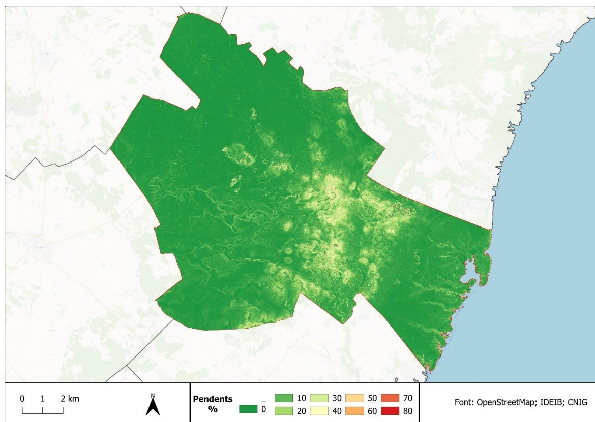
Figura 6. Mapa de pendents en percentatge del municipi de Felanitx. Font: Elaboració pròpia a partir de dades del CNIG.
