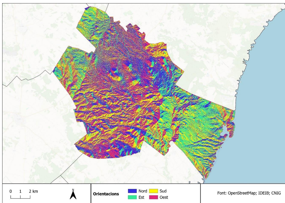
Figura 7. Mapa d'orientacions del municipi de Felanitx. Font: Elaboració pròpia a partir de dades del CNIG.
