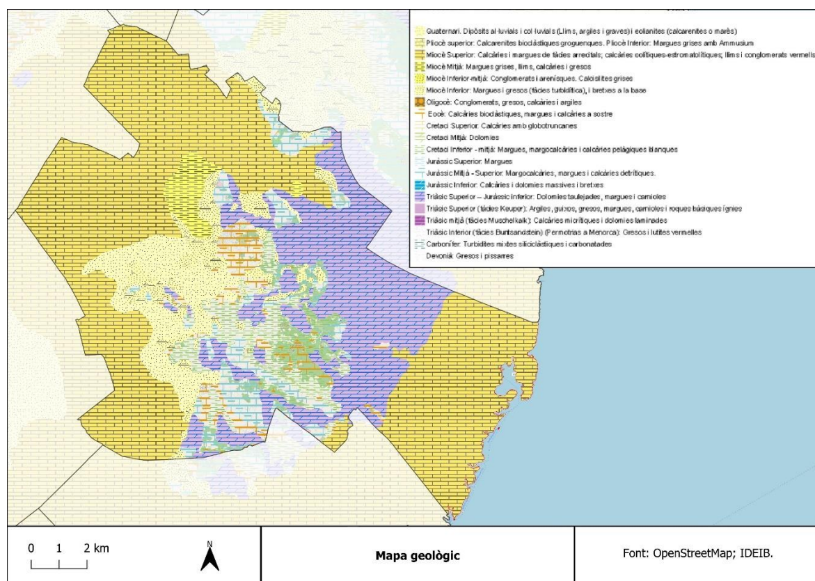
Figura 8. Mapa geològic del municipi de Felanitx. Font: Elaboració pròpia a partir de l'IDEIB.
